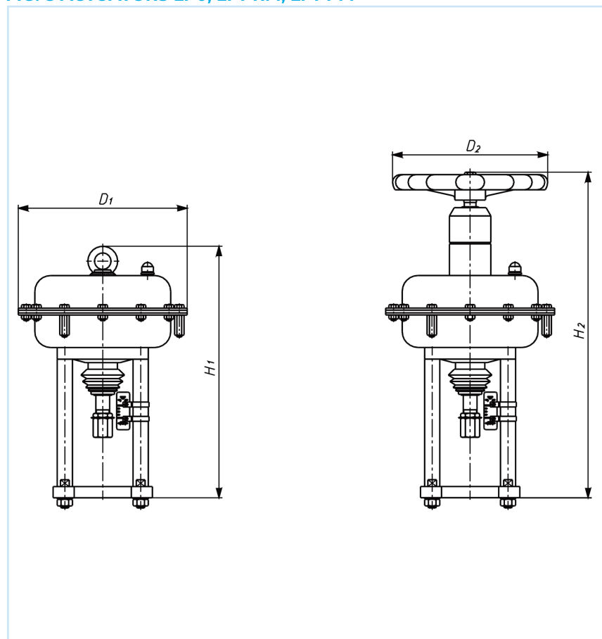
FIG. 8 ACTUATORS LP0, LP1-RM, LP1-PM
